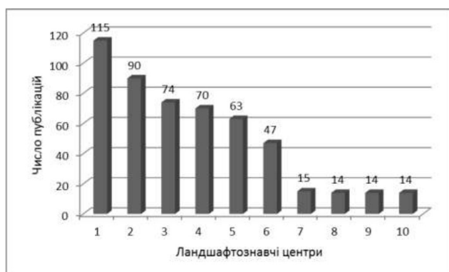
Рис. 3. Розподіл кількості публікацій між ландшафтознавчими центрами в 2001-2004 рр.: 1 – Львівський університет; 2 – Київський університет; 3 – Вінницький педуніверситет; 4 – Чернівецький університет; 5 – Інститут географії АН України; 6 – Таврійський університет; 7 – Тернопільський педуніверситет; 8 – Кіровоградський педуніверситет; 9 – Одеський університет; 10 – Сумський педуніверситет. (Міхелі, 2014).
