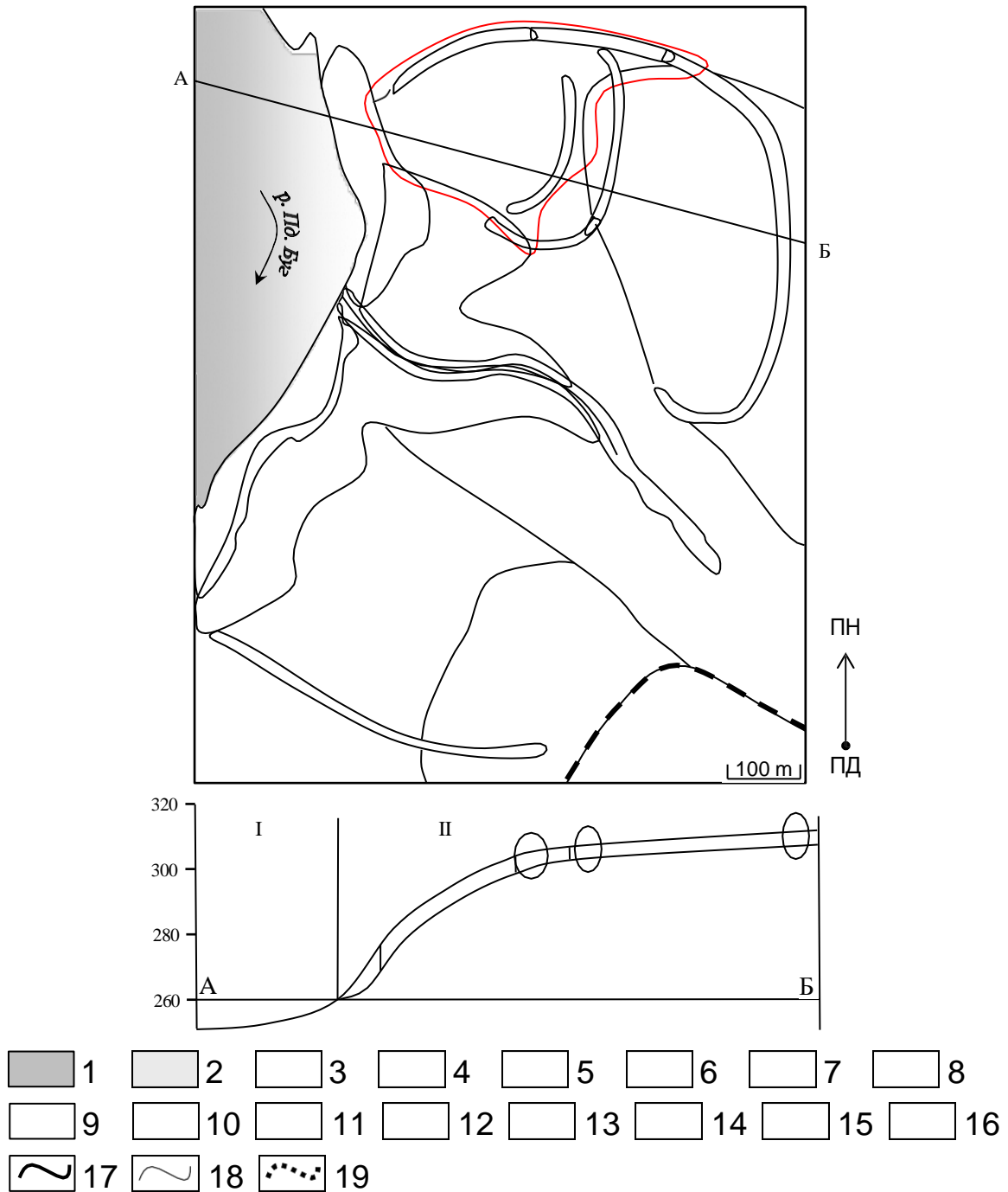
Рис. 1. Висотна диференціація та різноманіття белігеративних ландшафтів (Сабарівське городище)
