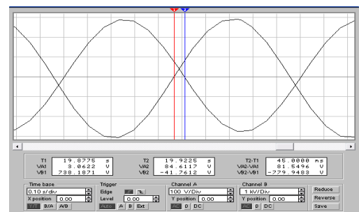
Рис. 3. Панель осцилографа з зображенням графіків змінних струмів двох генераторів.
